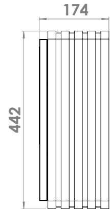
EVO60-RIB
